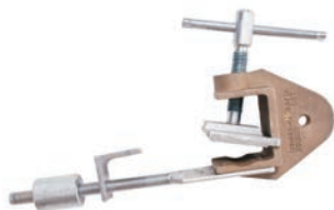
CLEMA DE LEGARE LA ȘINA DE CALE FERATĂ
